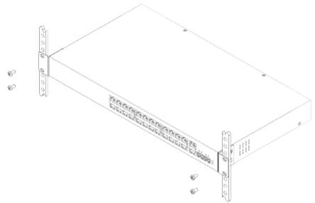
제품을 랙에 설치하는 방법
