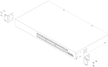
제품에 브라켓을 설치하는 방법
