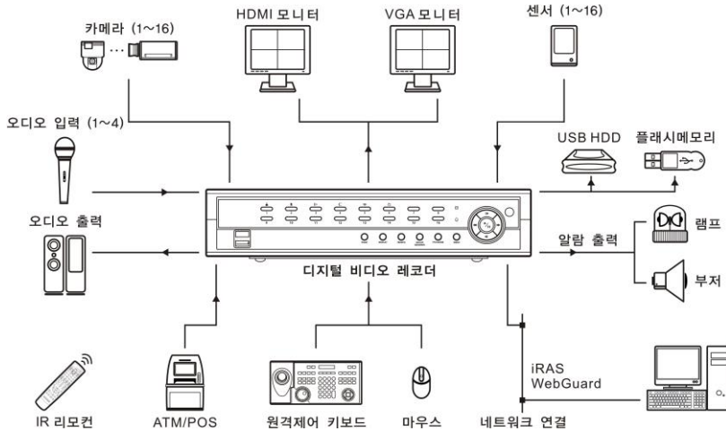
그림 1: 샘플구성도
