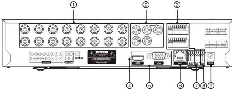
그림 2: DVR 후면 패널
