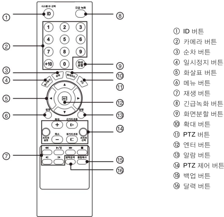
그림 4: IR 리모컨
