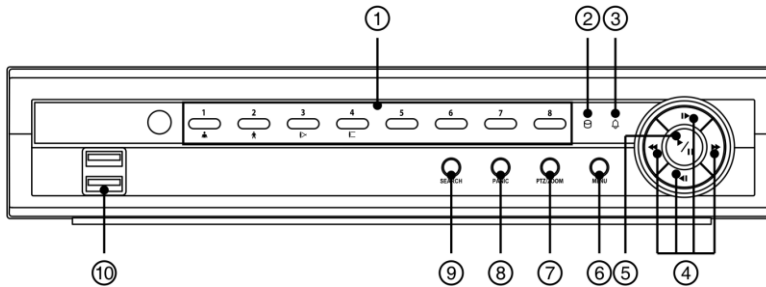
그림 3: 8채널 DVR 전면 패널
