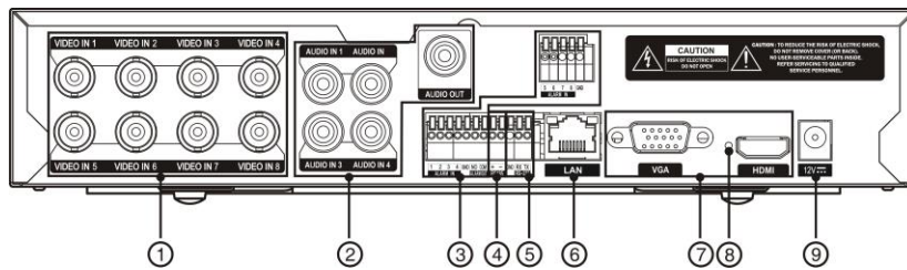
그림 2: 8채널 DVR 후면 패널
