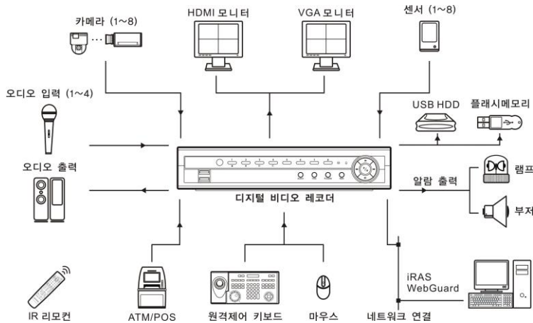
그림 1: 샘플구성도
