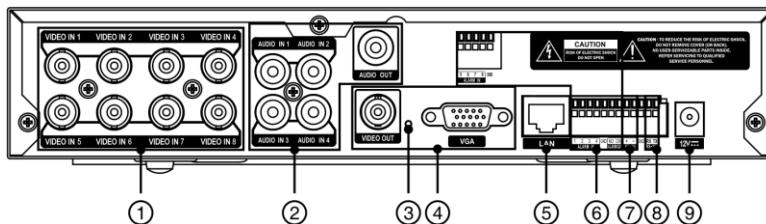
그림 2 — 8채널 DVR 후면 패널
