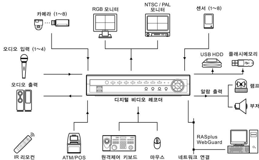
그림 1 — 샘플구성도
