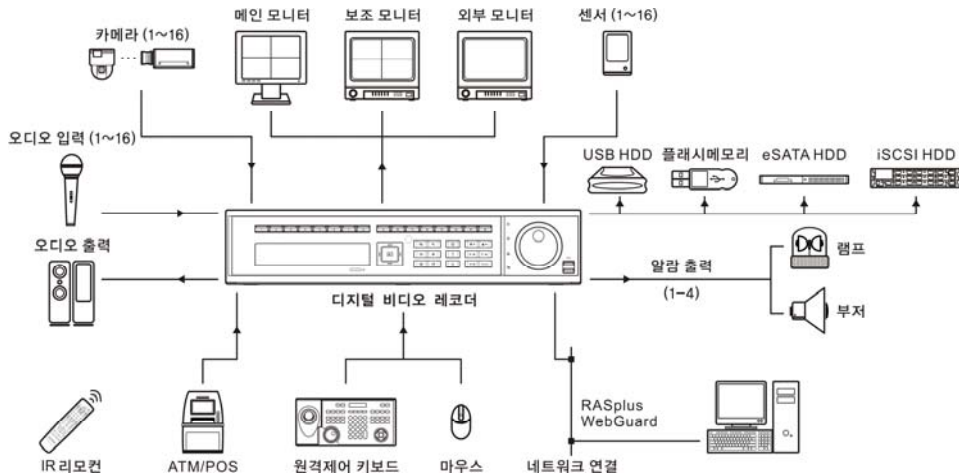
그림 1: 샘플구성도
