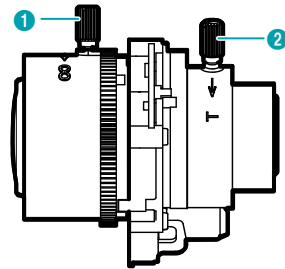
가변 초점 자동 조리개 렌즈
