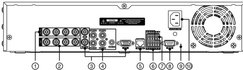
그림 2 — DVR 후면 패널
