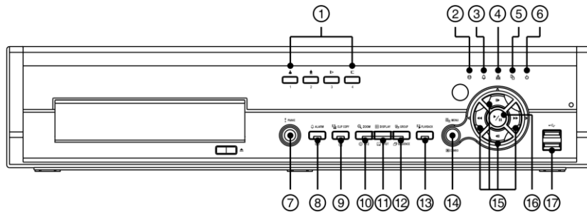
그림 3 — DVR 전면 패널
