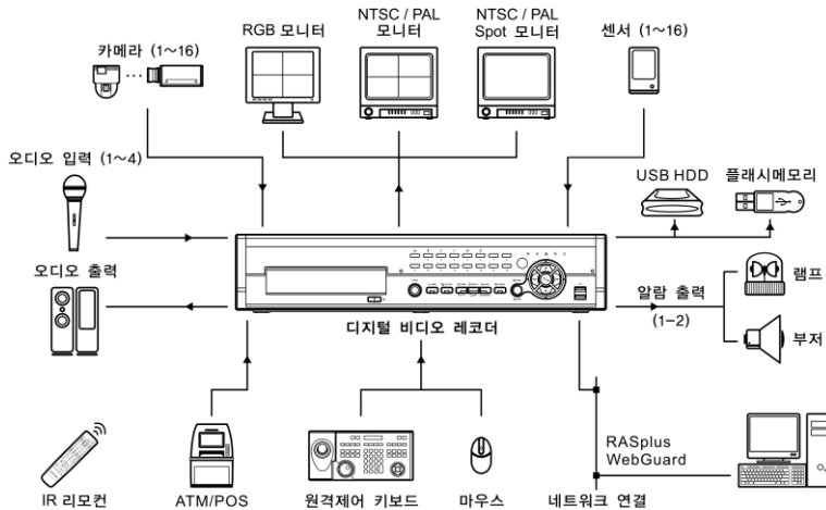
그림 1 — 샘플구성도
