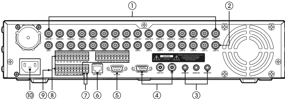
그림 2—16 채널 DVR 후면 패널
