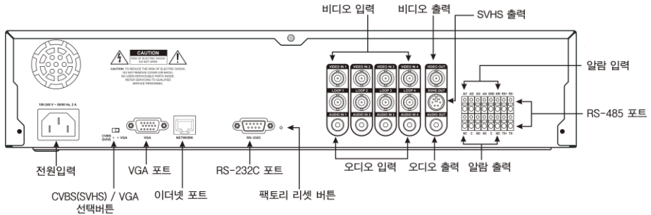
그림 2 — DVR 후면 패널
