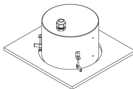
매립형 (MNC221SF 모델)
