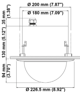
매립형 (MNC221SF 모델)
